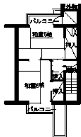
2階平面図
