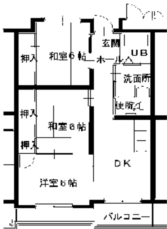
<3DK>
