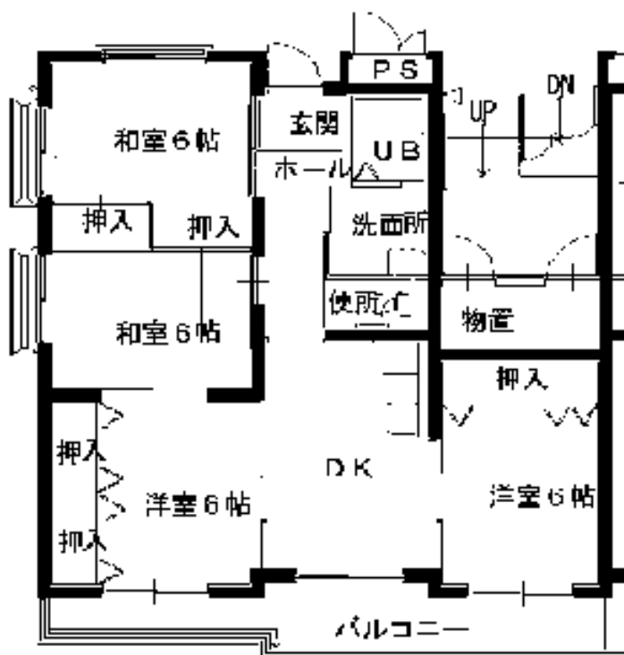
<4DK>
